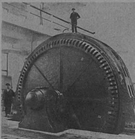
3600 K.V. A. Kolmivaihegeneraattori.
