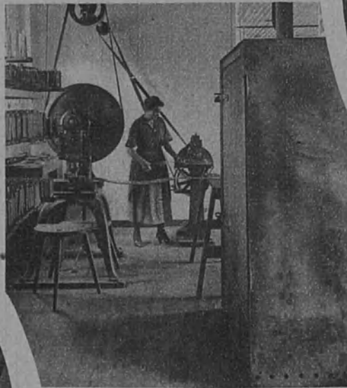
Valssatut lyijy- tai linaharkot saksataan ja senjälkeen lyödään niistä tuubin läpimitää vastaavat lanlit. Kuvassa oikealla kuivauskaappi värinpainetuille tuubeille. — Oikealla: Muutamia Oy. Hermetic Ab:n valmistamia tuubeja.
